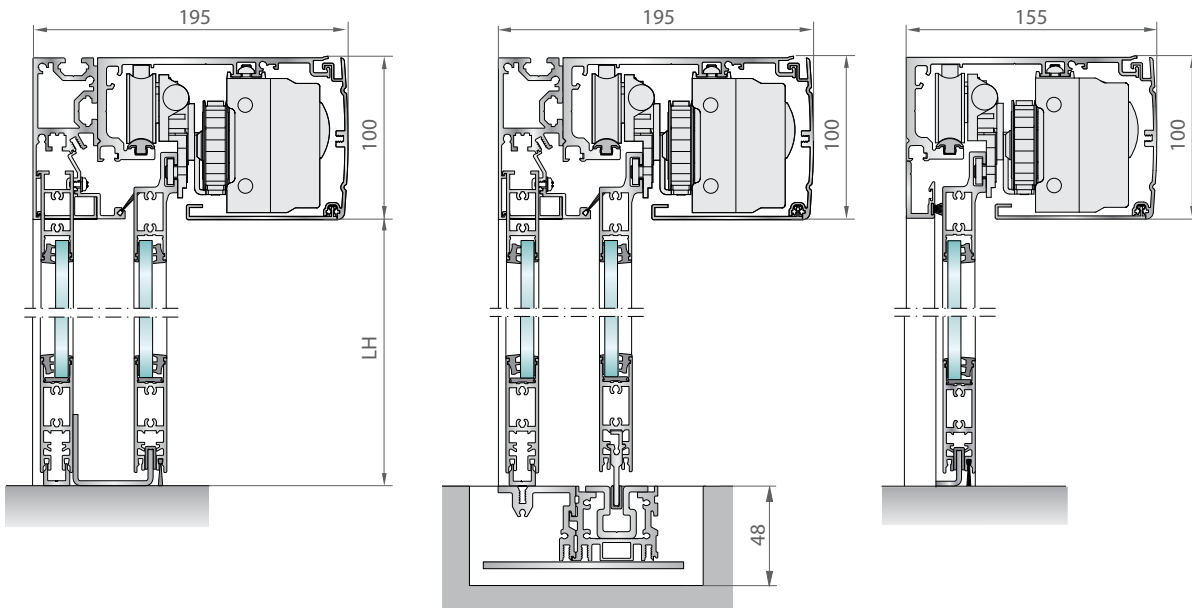
Una y dos hojas correderas Una y dos hojas fijas con guía estándar
